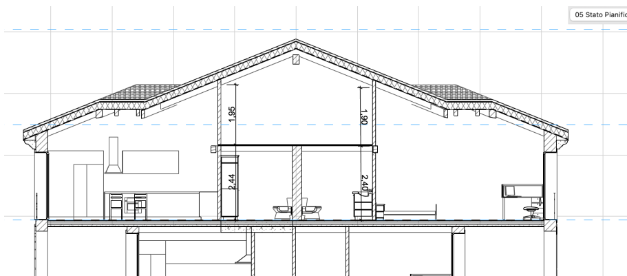
Sezione
