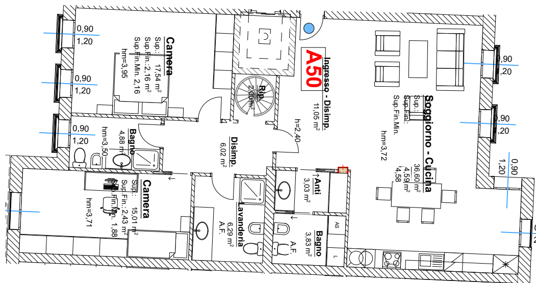
Appartamento 50 - Pianta Piano Secondo
