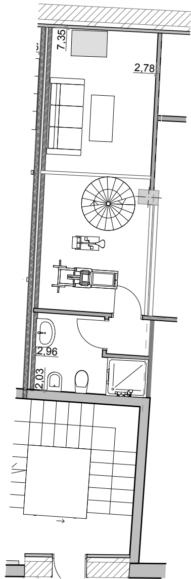
Soppalco 1:100
