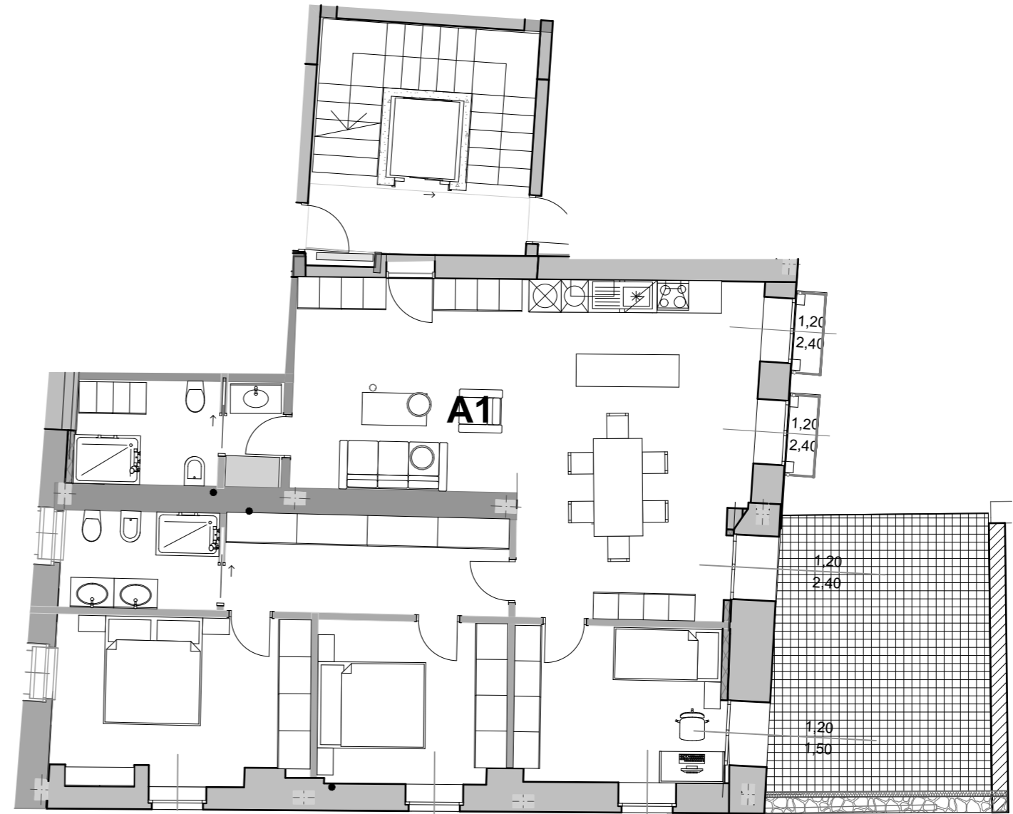
1. Pianta Piano Primo 1:100
